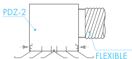
Montage aan plenum
