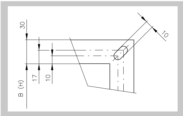
Fig. 9 Flange
