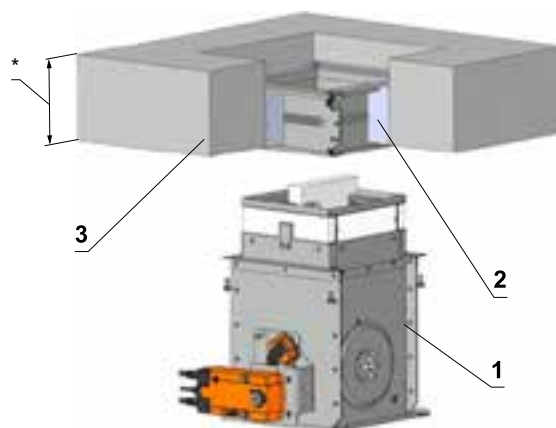
Installation frame E2
