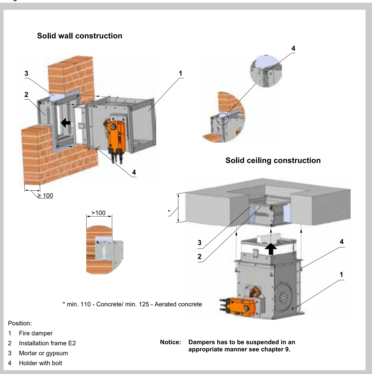
Fig. 75 Installation frame E2
